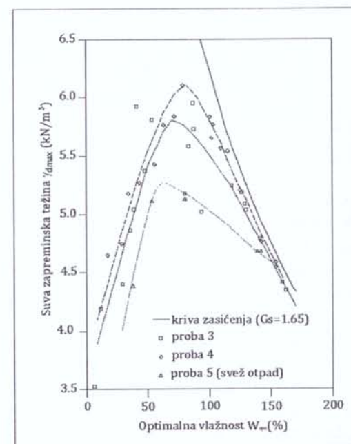
Slika 3. Krive zbijanja za korišćen otpad (Hettiarachchi, 2005) [4]
