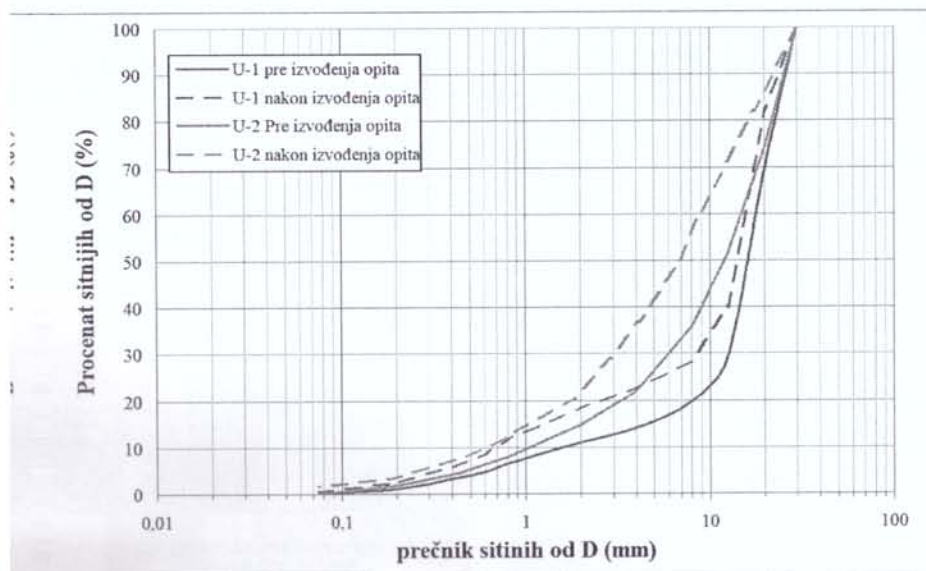
Slika 9. Granulometrijske krive pre i nakon izvođenja Proktorovog opita (malj sa šiljcima)
