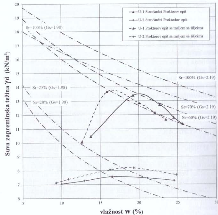
Slika 10. Prikaz rezultata istraživanja Proktorovog opita (standardni malj i malj sa šiljcima)
